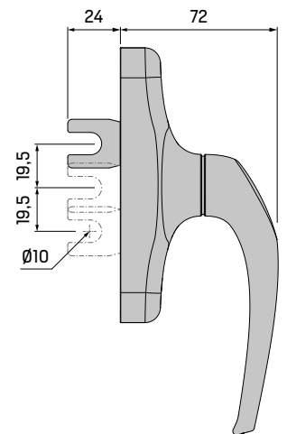
■ APERTURA OSCIOBATIENTE TILT & TURN OPENING
